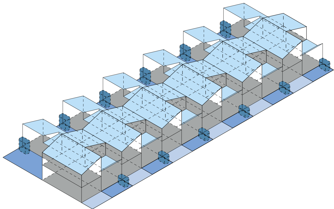
axo (landscape)
